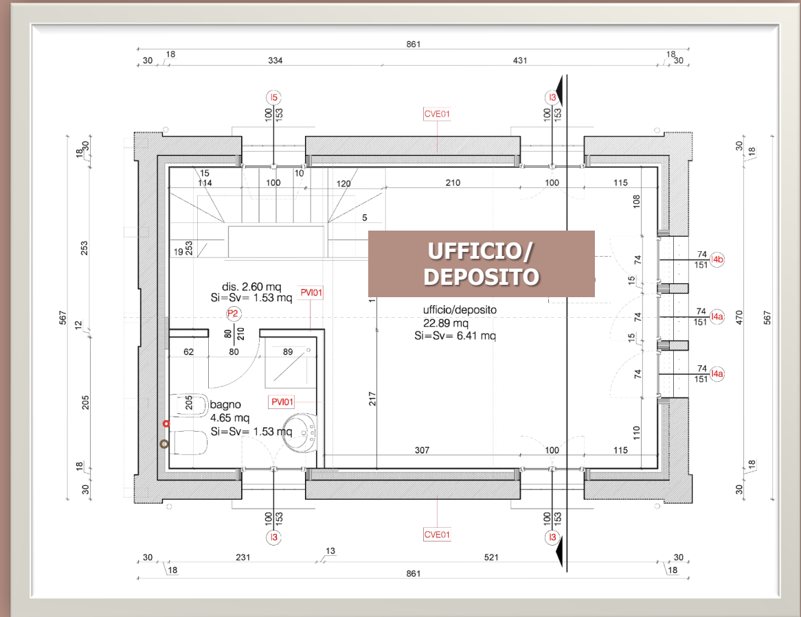
PIANO PRIMO superficie lorda 50 mq
