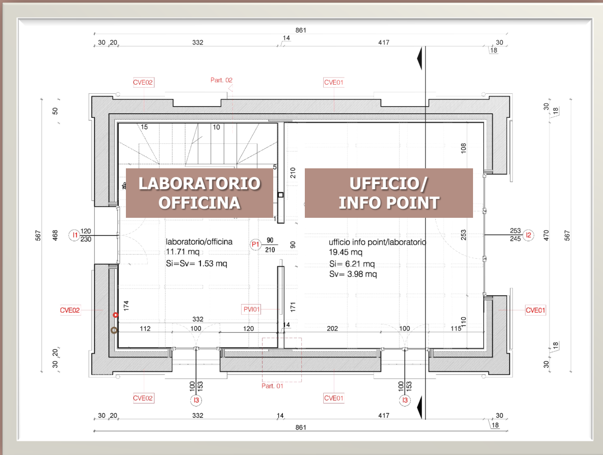
PIANO TERRA superficie lorda 50 mq
